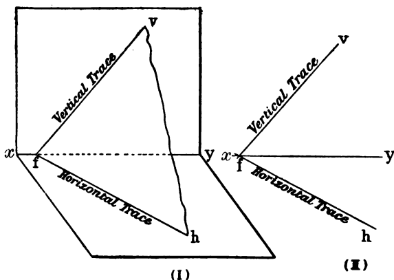
FIG. 94.—Oblique Plane.
