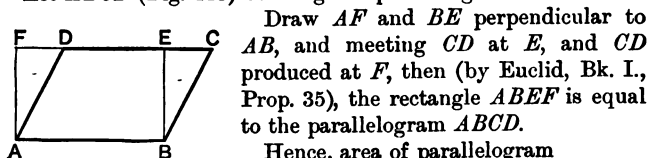
FIG. 113.—Area of a parallelogram.
