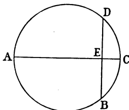
FIG. 29.— AE \times EC = BE^2 .
